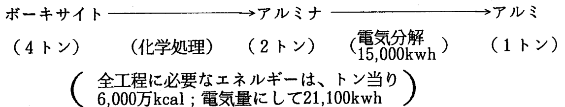
図1. アルミの製錬工程と必要エネルギー量
